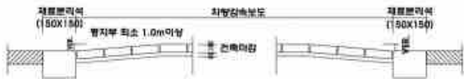
차량감속보도 횡단면도
